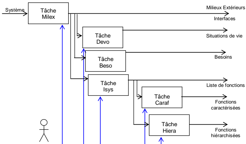
Figure 10 — Actigramme SADT d'une AF externe.
