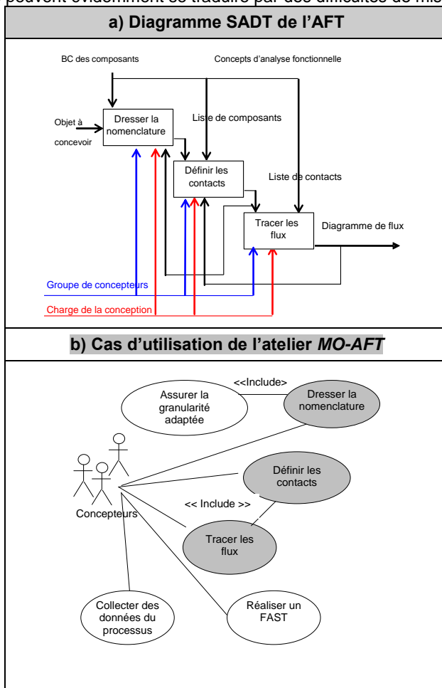
Figure 13 — Diagramme SADT des premières phases de l'AFT et cas d'utilisation pour leur instrumentation.
