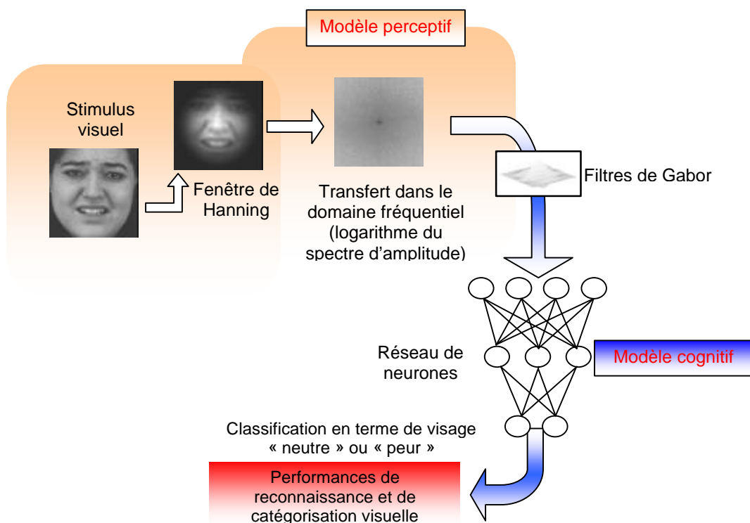
Figure 1 — Couplage des modèles computationnel et connexionniste.
