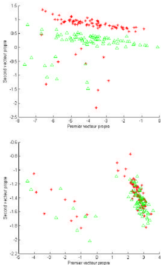
Figure 4 — Distribution statistique des stimuli par projection sur l'espace plan composé des 2 premiers vecteurs propres.
