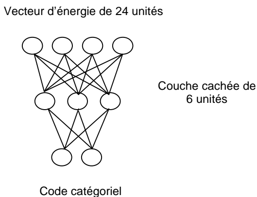
Figure 3 — Architecture du réseau connexionniste.
