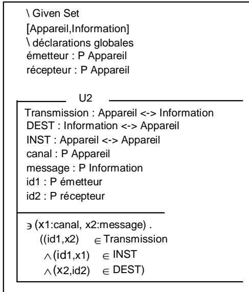
Figure 6 — Traduction en Z du graphe conceptuel u .
