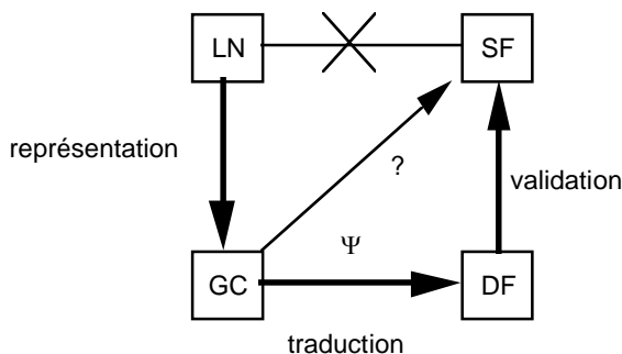
Figure 3 — Synthèse schématique des 3 hypothèses (LN : Langage Naturel; GC : Graphe Conceptuel; DF : Description Formelle; SF : Spécification Formelle; LP : Logique des Prédicats; Y=f \circ f' ; f : GC \rightarrow LP ; f' : LP \rightarrow DF )
